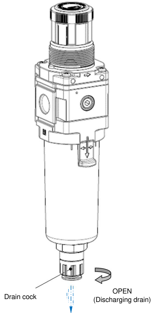
AWD30-D/ AWD40-D: Auto drain
