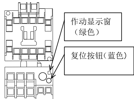
热继电器
