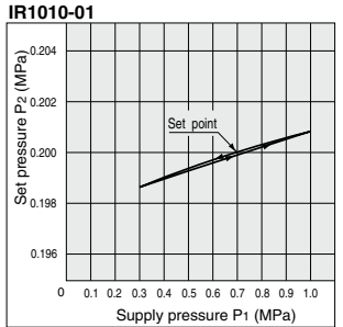
IR1010-01 Back pressure: 0.7 MPa
